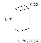
Pensili H. 70
