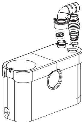
Рис. 5 Напорный патрубок
