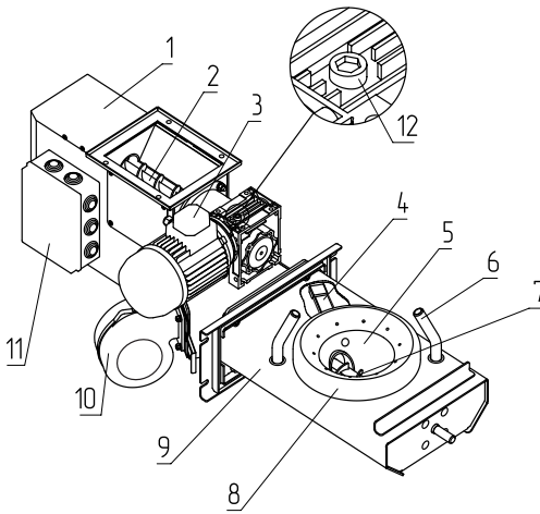
Рис.4. Pelletная горелка с приводом.
