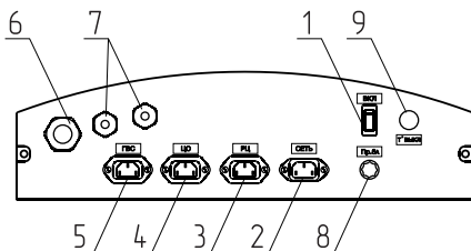
Рис.6. Расположение органов управления на задней панели пульта.
