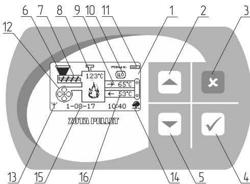
Рис.5. Расположение органов управления и индикации на передней панели пульта.
