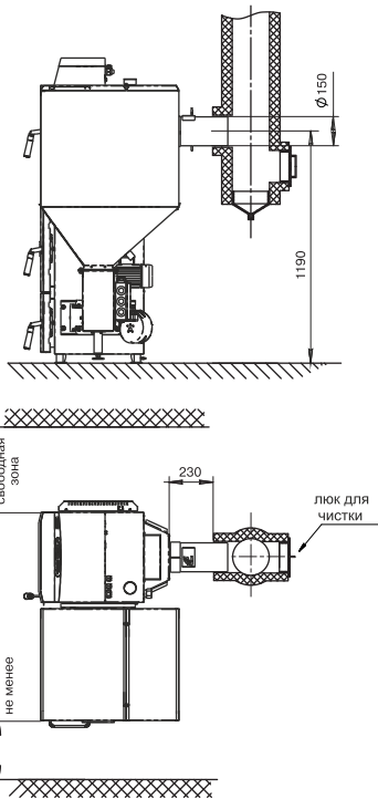
Рис.7. Схема установки котла.
