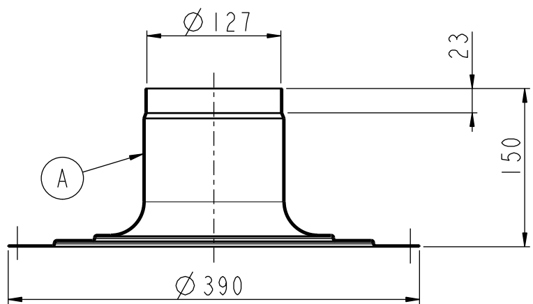
SEZIONE A-A
