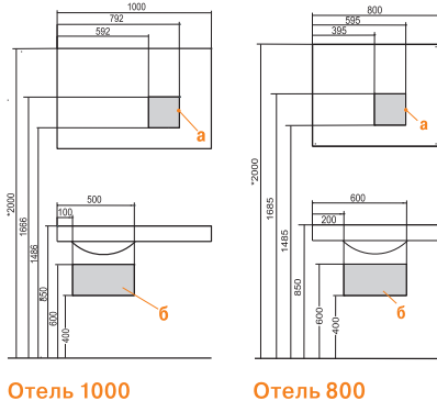
Схема подключения:
