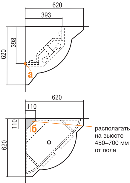
Схема подключения:
