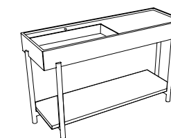
PLINIO 140 con piano Plinio 140 с полочкой столешница cm 140 x 46 x 82,5 h P. 150
