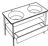
CATINO DOPPIO con cassetto Catino Doppio с ящиком cm 110 x 58,5 x 83 h P. 142
