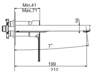
SPOUT 200 MM - ИЗЛИВ 200 MM
