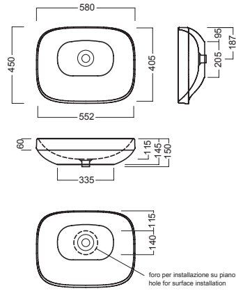
lavabo 80 washbasin 80
