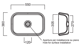
lavabo 55 washbasin 55
