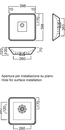
lavabo 10:00 washbasin 10:00
