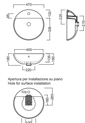
lavabo 03:00 washbasin 03:00
