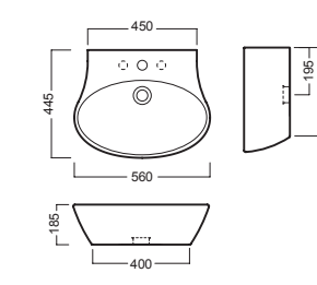
lavabo 56 washbasin 56
