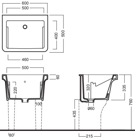
lavatoio 60 sink 60
