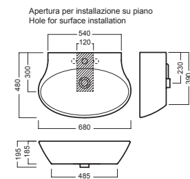
lavabo 68 washbasin 68
