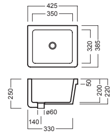
lavatoio 38 sink 38
