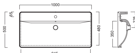
lavabo 100 washbasin 100
