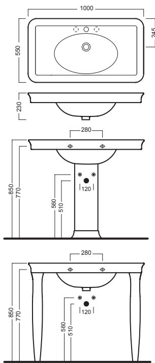
lavabo 100 washbasin 100
