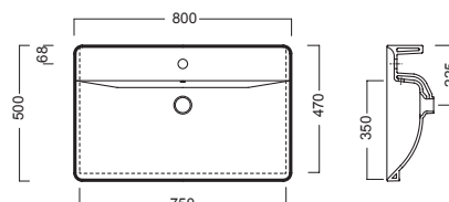
lavabo 80 washbasin 80
