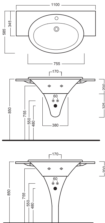
lavabo 110 washbasin 110
